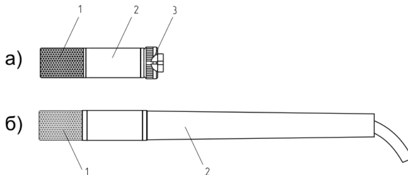
Рисунок 3.10 Измерительные преобразователи
