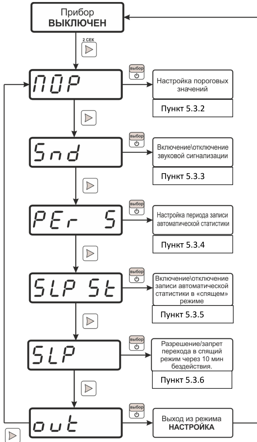
Рисунок 5.6 Схема режима НАСТРОЙКА ИВТМ-7 М 2(-Д), ИВТМ-7 М 5(-Д)
